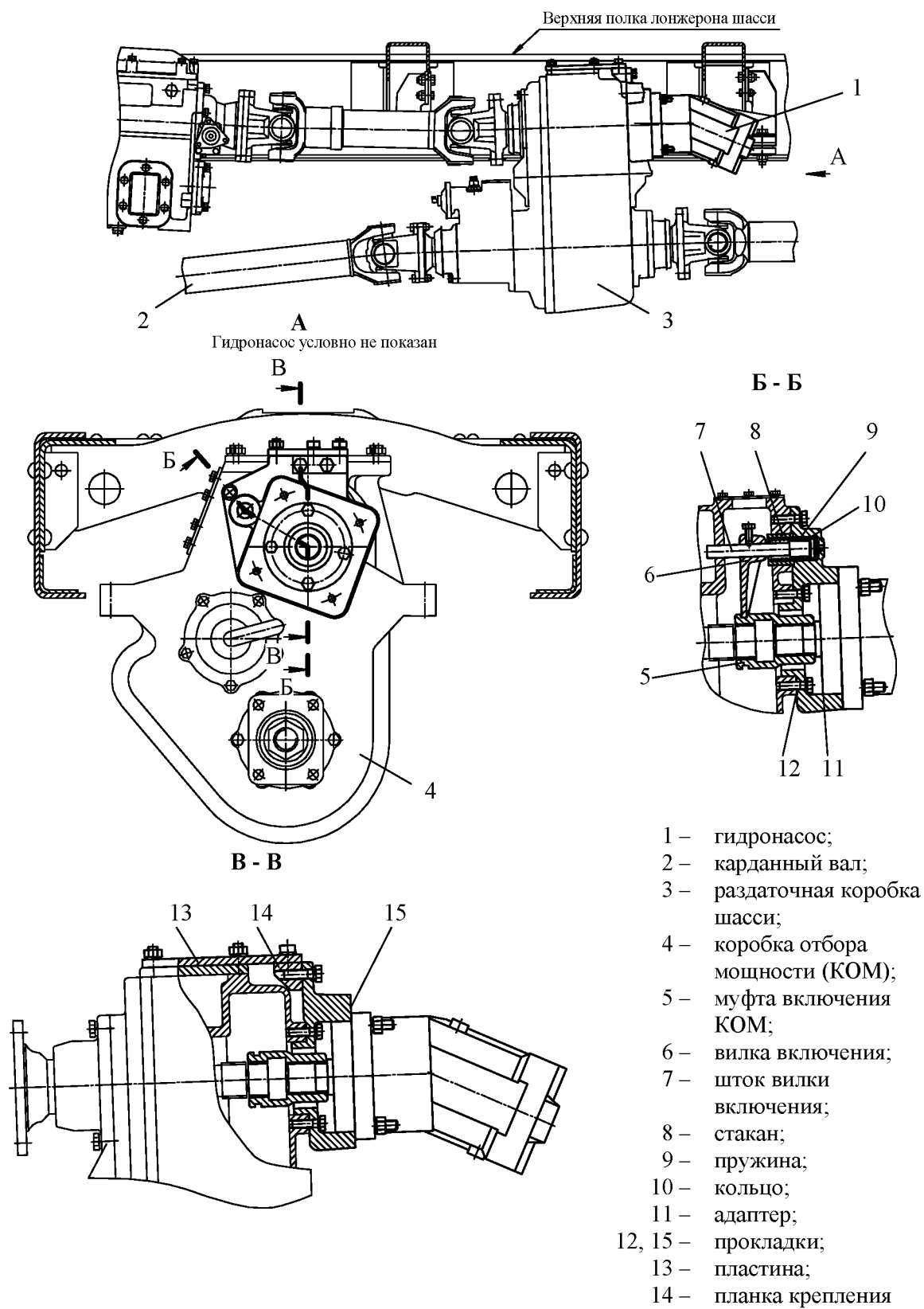
Рисунок 2.6 – Привод насоса
