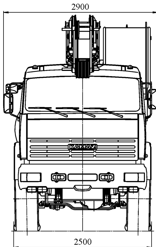
Рисунок 1.2 – Общий вид крана в транспортном положении спереди
