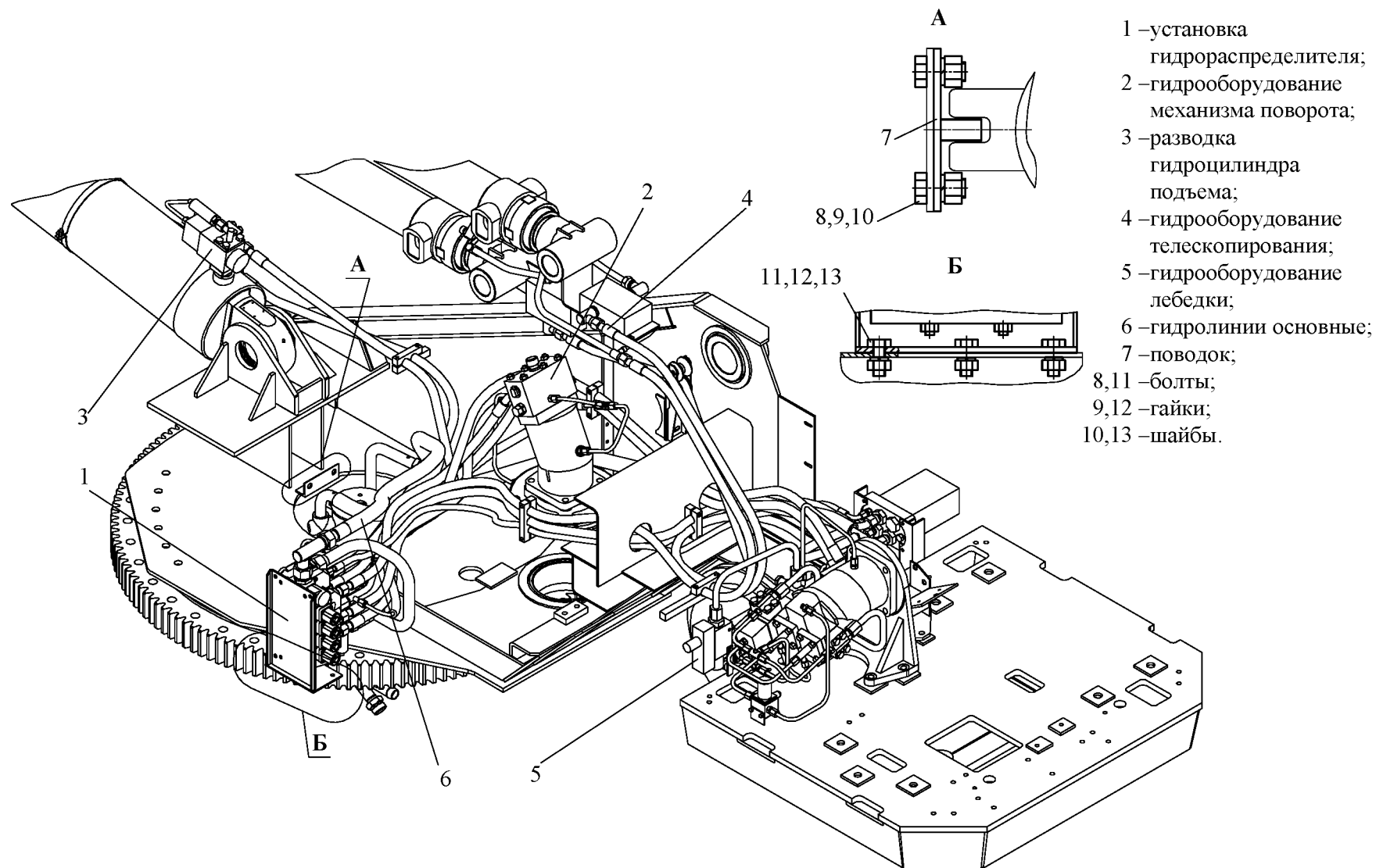
Рисунок 4.31 – Гидрооборудование поворотной части
