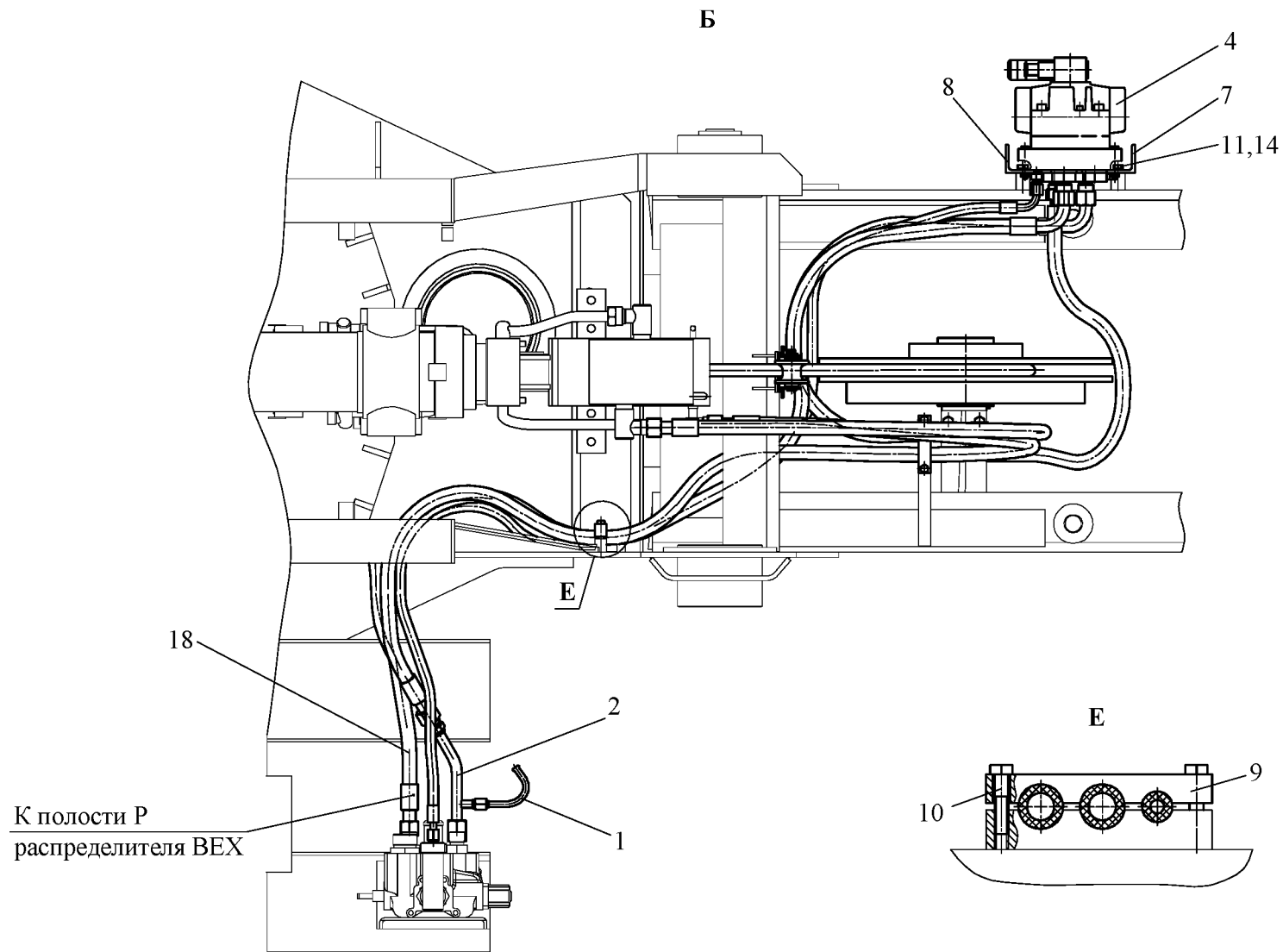
Рисунок 4.37.2 – Гидрооборудование телескопической стрелы
