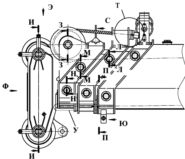
Рисунок 3.17.2 - Стрела телескопическая
