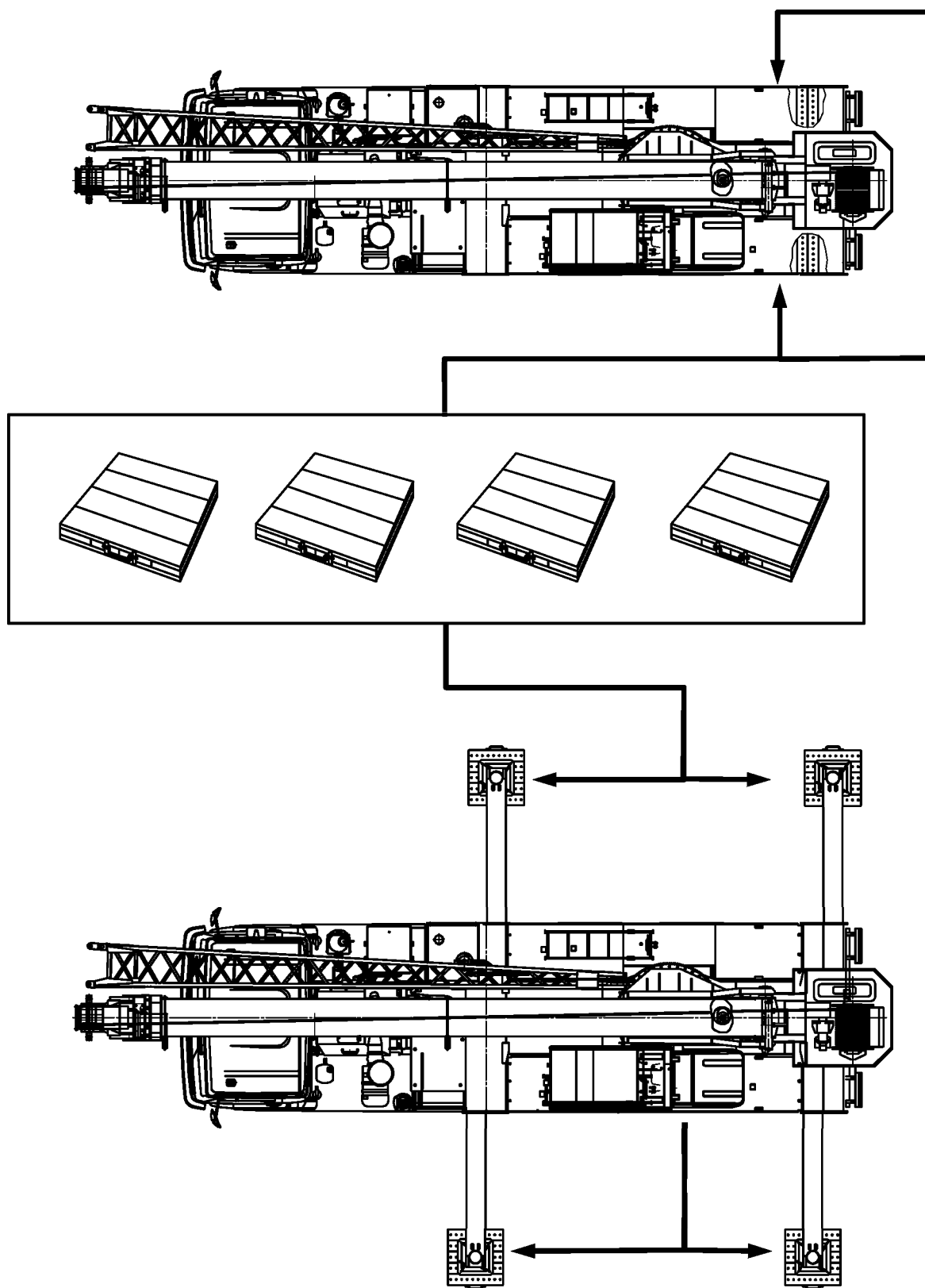
Рисунок 2.8 – Размещение инвентарных подкладок в транспортном и рабочем положениях крана
