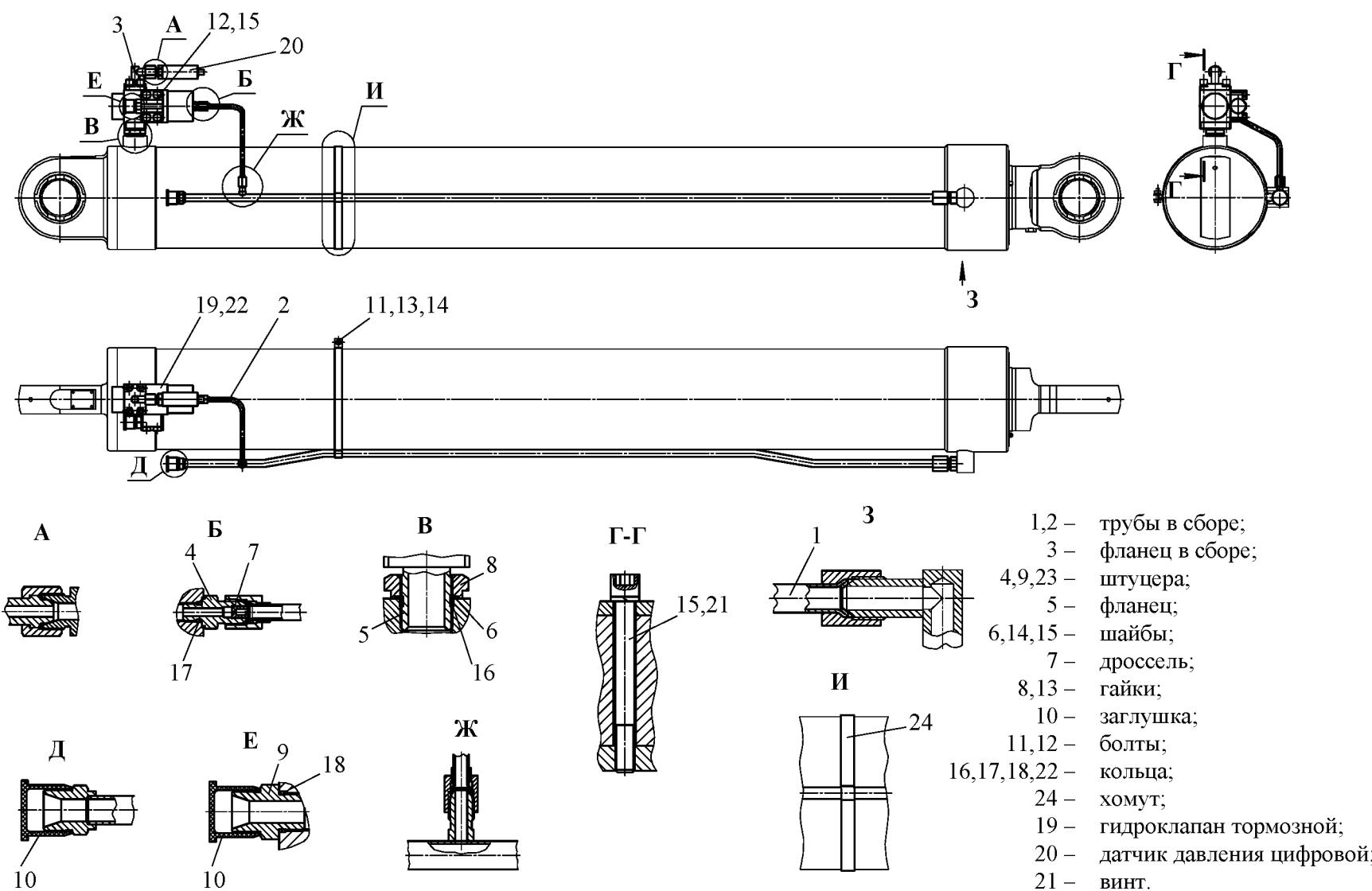
Рисунок 4.36 – Разводка гидроцилиндра Ц-200.200.00.000
