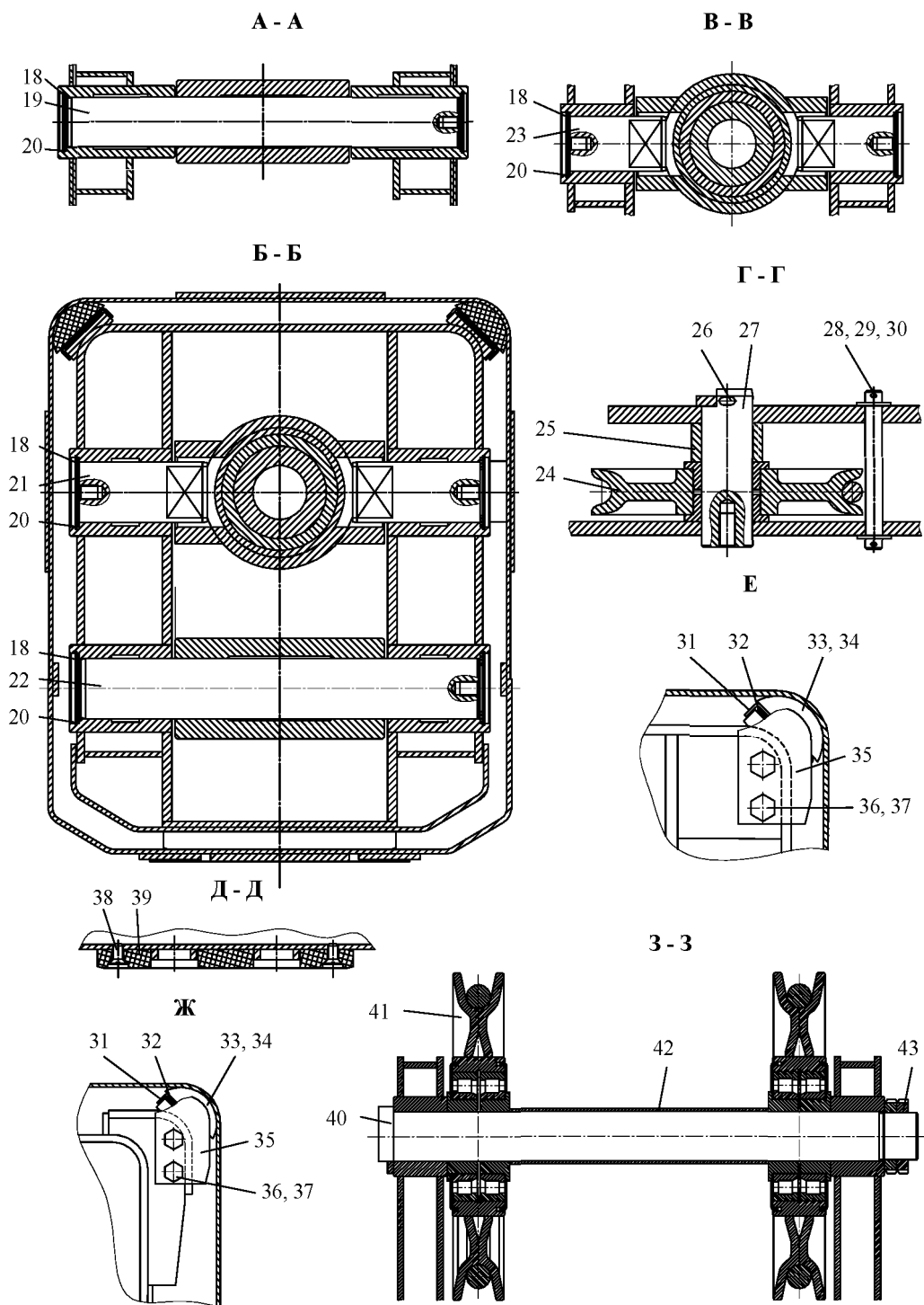
Рисунок 3.17.3 - Стрела телескопическая
