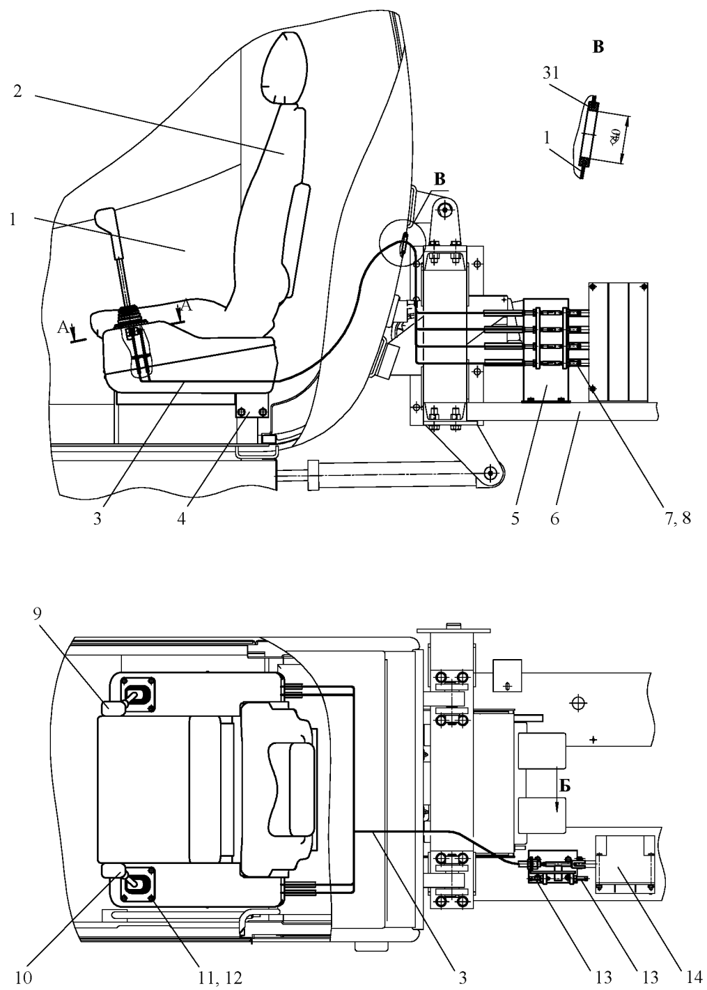
Рисунок 3.22 – Схема приводов
