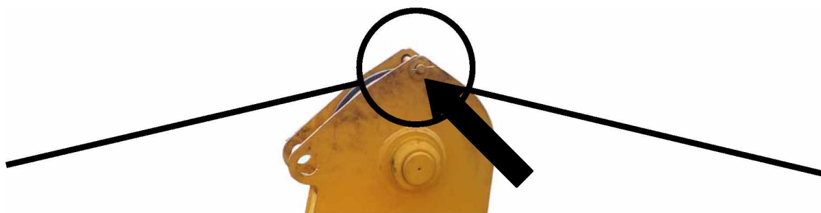
Рисунок 13.19 – Установка оси на блоке основания гуська
