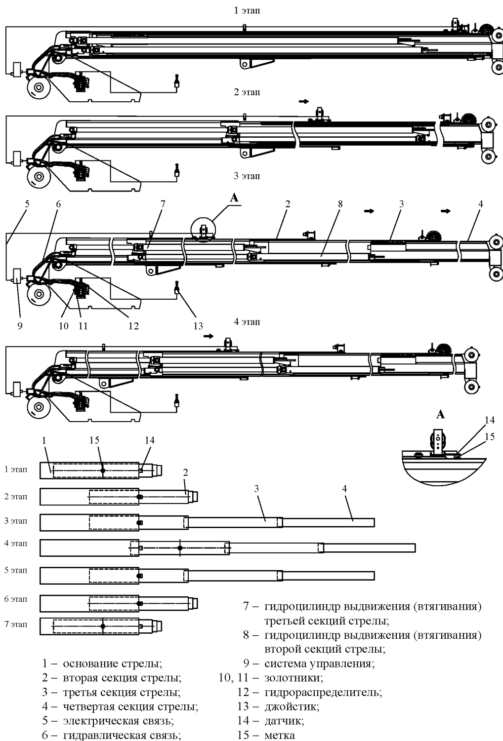
Рисунок 3.18 – Схема телескопирования стрелы
