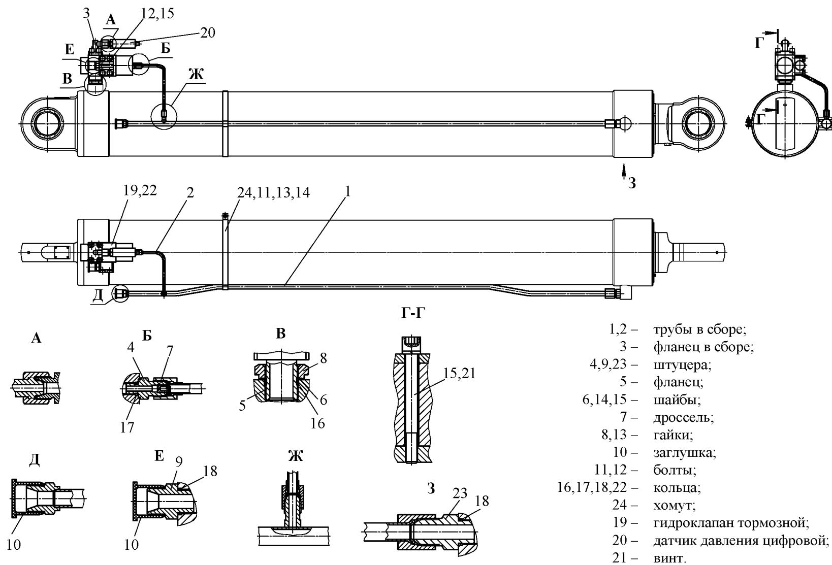
Рисунок 4.35 – Разводка гидроцилиндра КС-45717.63.400-5
