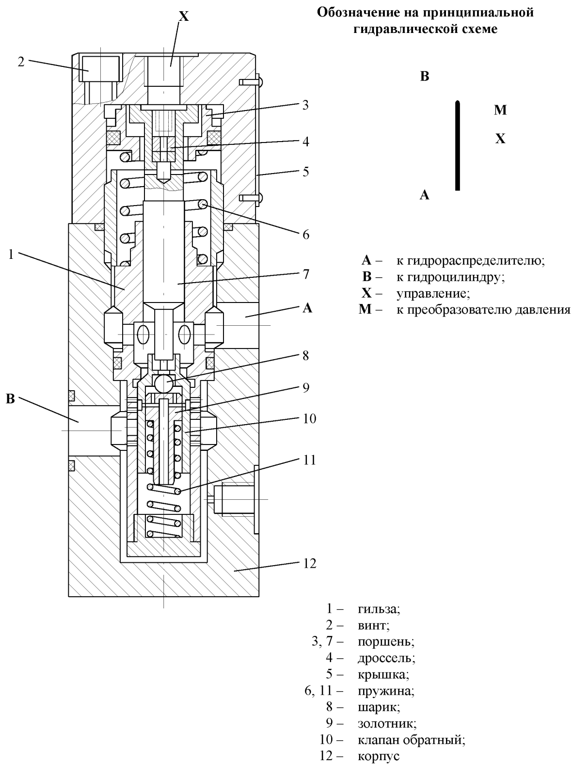
Рисунок 4.19 – Клапан тормозной механизма изменения вылета
