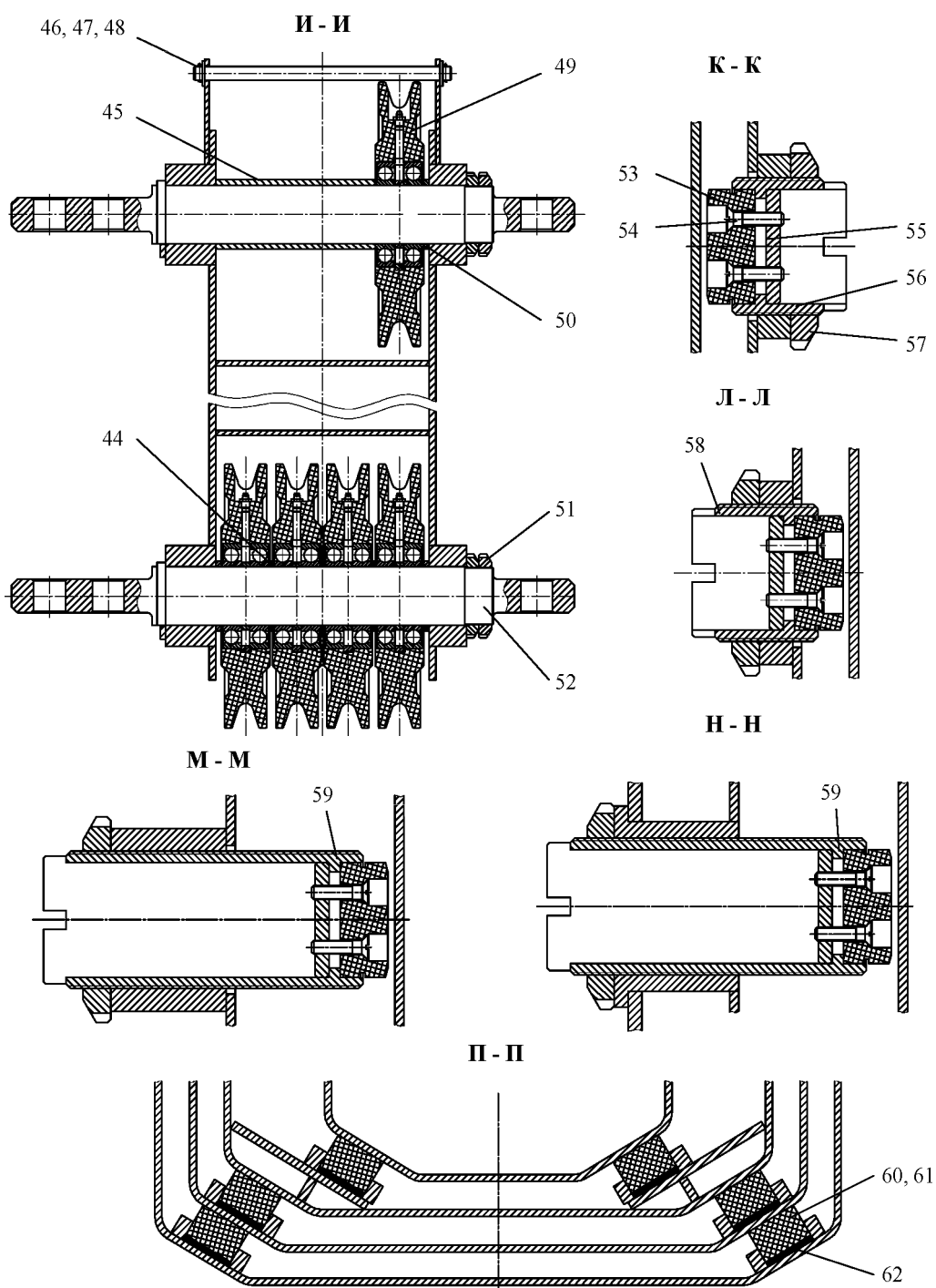
Рисунок 3.17.4 - Стрела телескопическая
