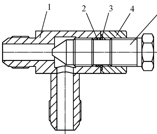
Дроссель ДР6
