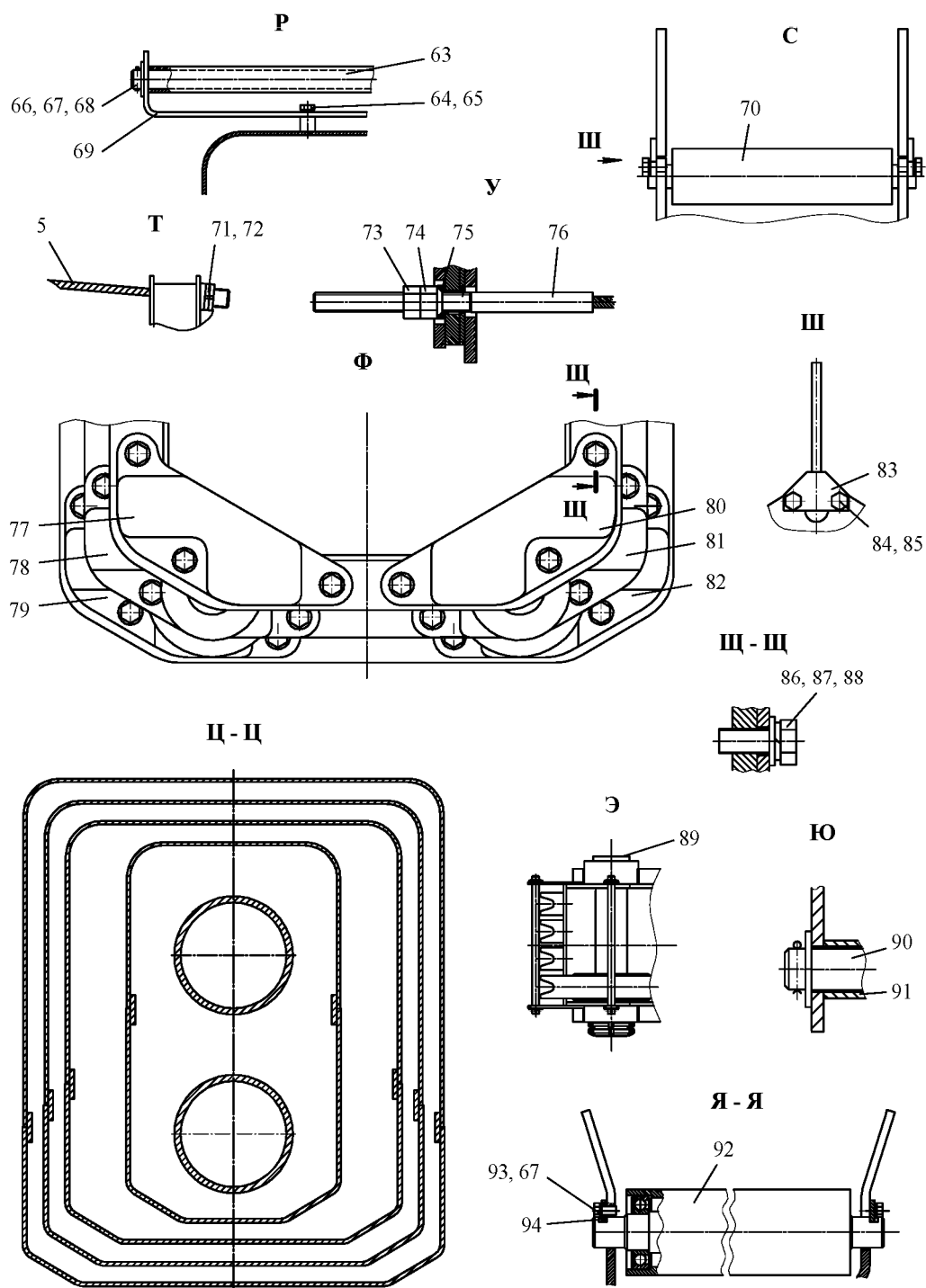
Рисунок 3.17.5 - Стрела телескопическая
