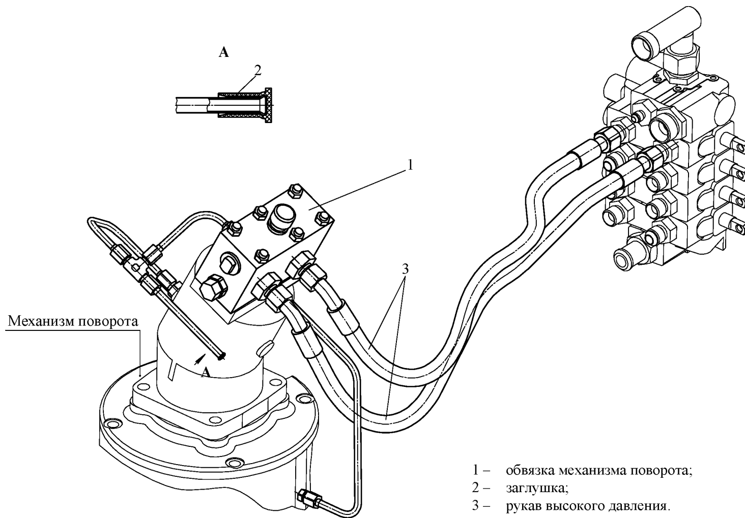
Рисунок 4.32 – Гидрооборудование механизма поворота
