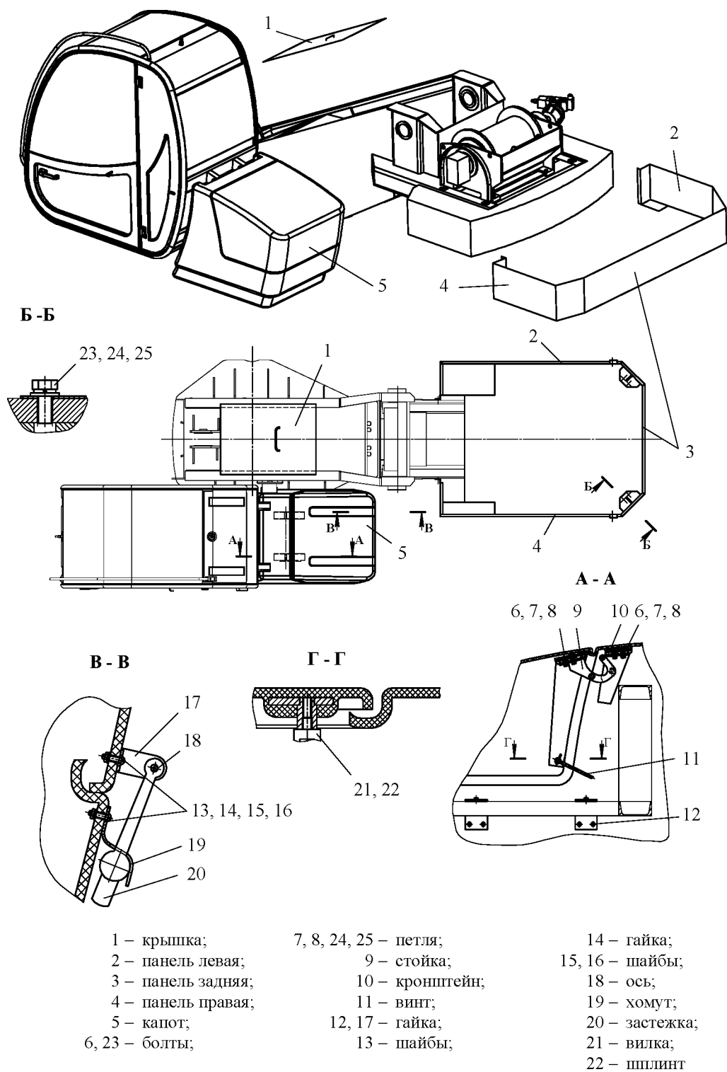
Рисунок 3.2 – Кожухи
