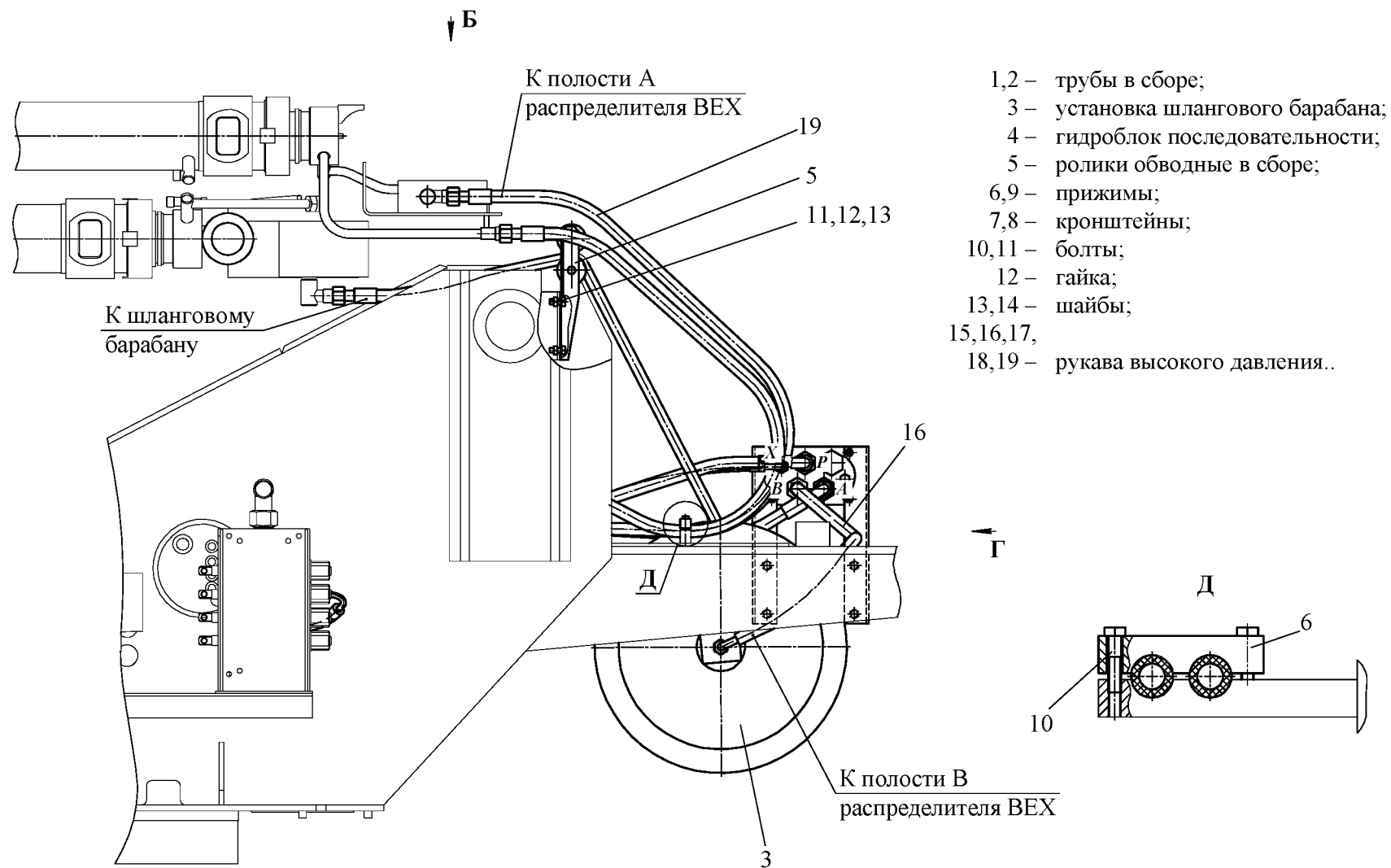
Рисунок 4.37.1 – Гидрооборудование телескопической стрелы
