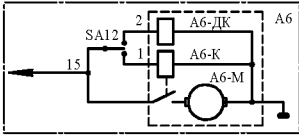
А6 Установка подъема (опускания) кабины
