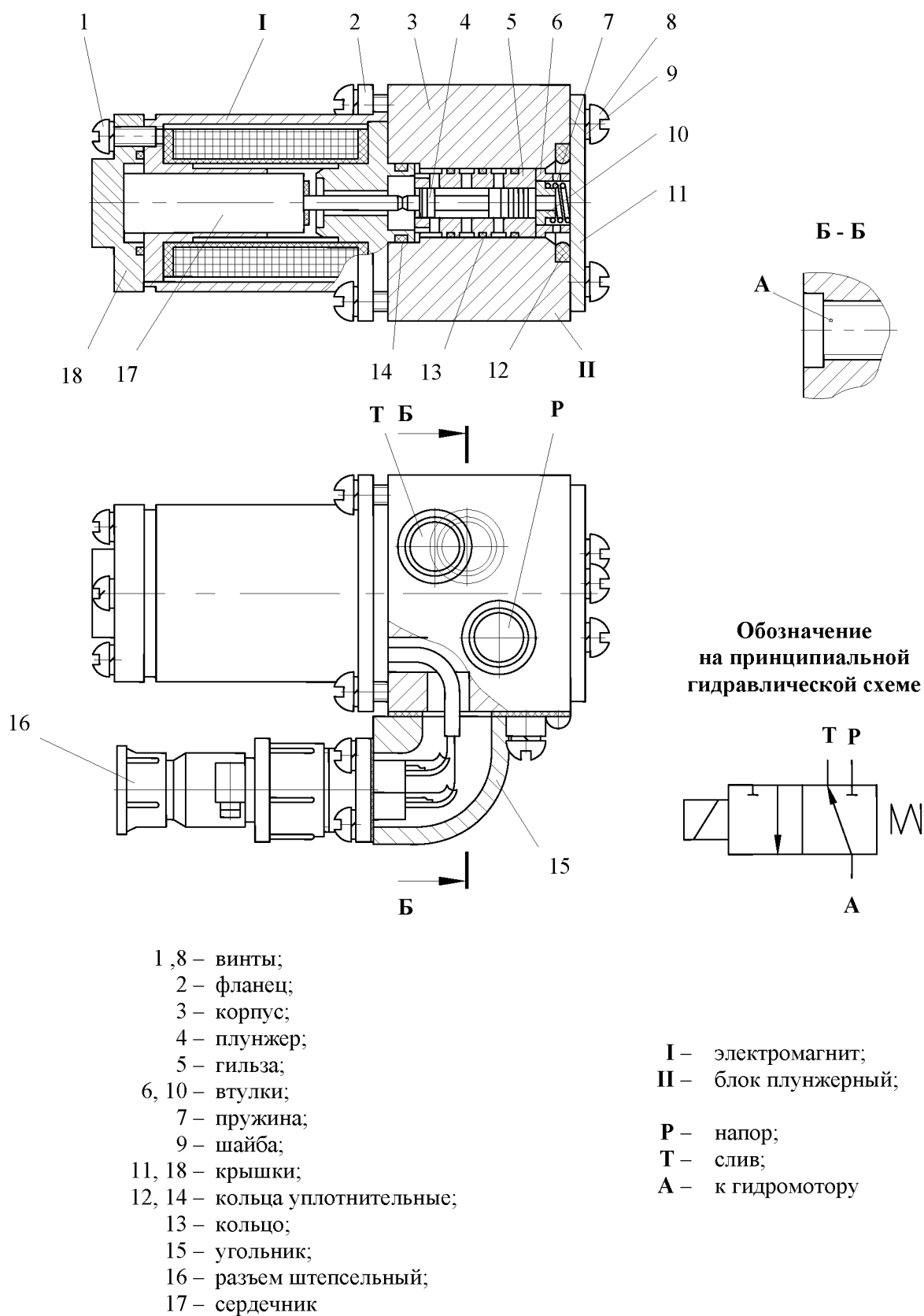
Рисунок 4.8 - Гидрораспределитель с электрическим управлением
