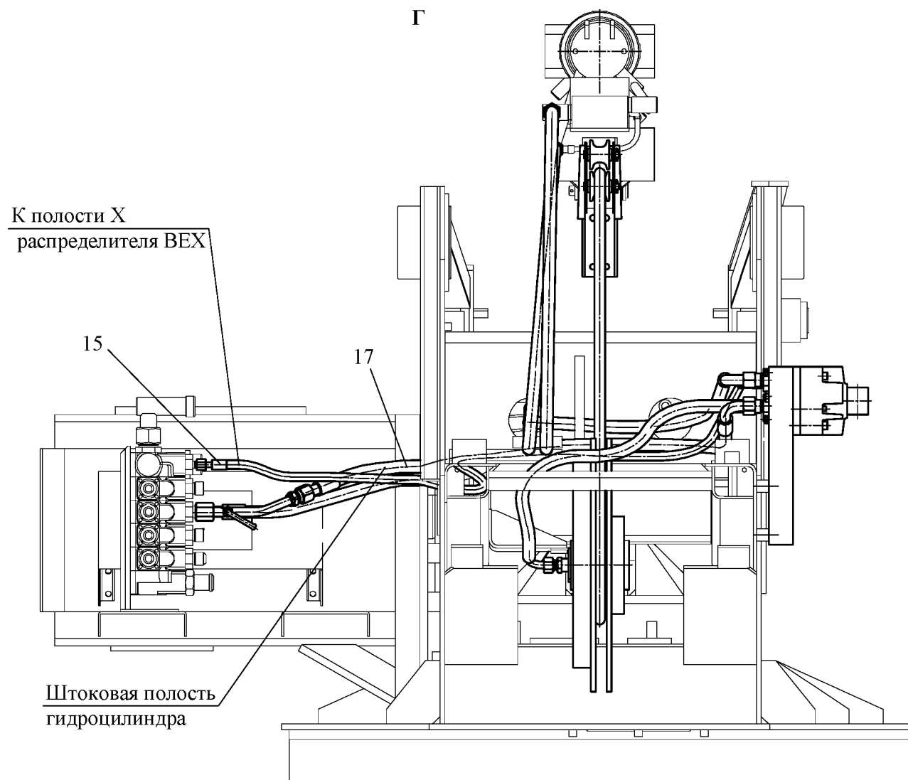
Рисунок 4.37.3 – Гидрооборудование телескопической стрелы
