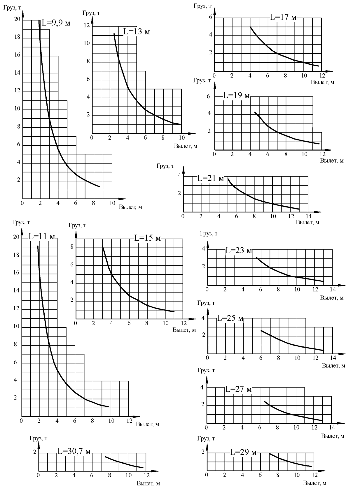
Рисунок А.3 – Грузовые характеристики крана на втянутых выносных опорах в зоне работы 220^\circ
