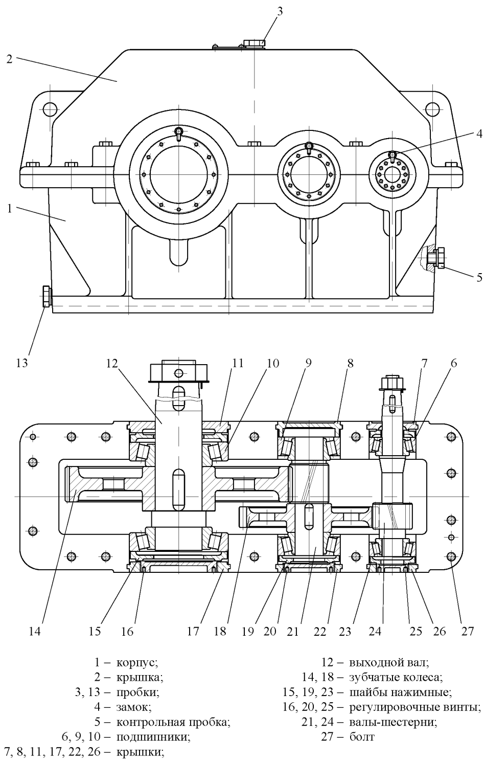
Рисунок 3.12 – Редуктор
