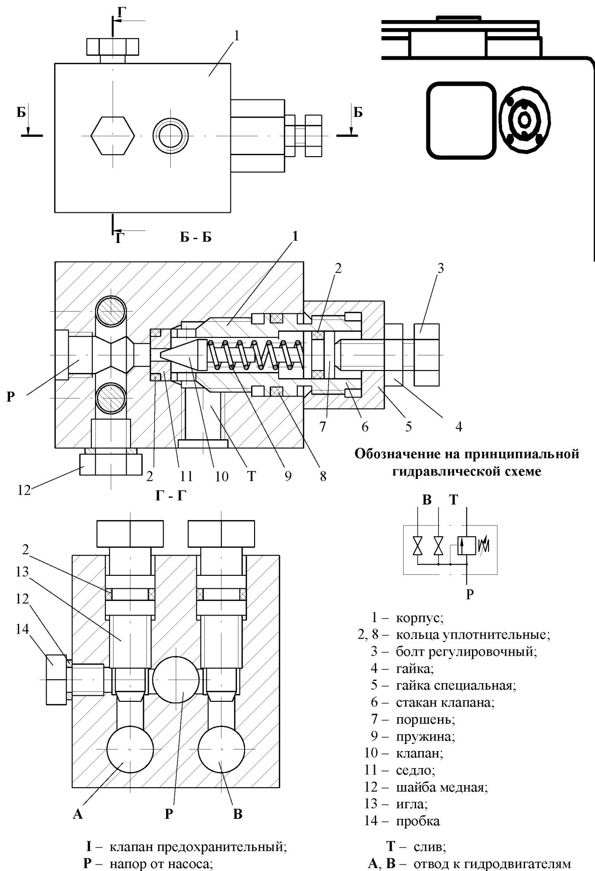
Рисунок 4.25 – Гидроблок аварийный
