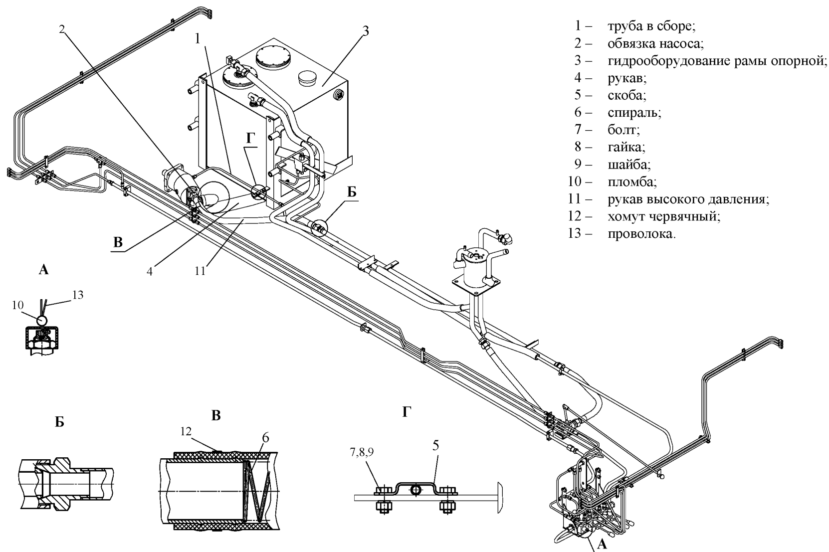
Рисунок 4.30 – Гидрооборудование неповоротной части
