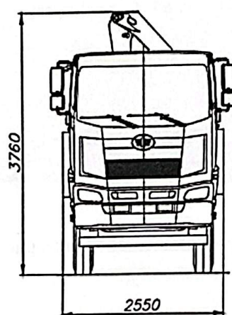
Рис.3. Геометрические параметры крана-манипулятора
