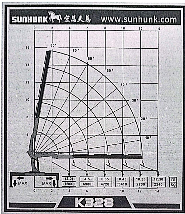
Рис.2. Грузовысотные характеристики.
